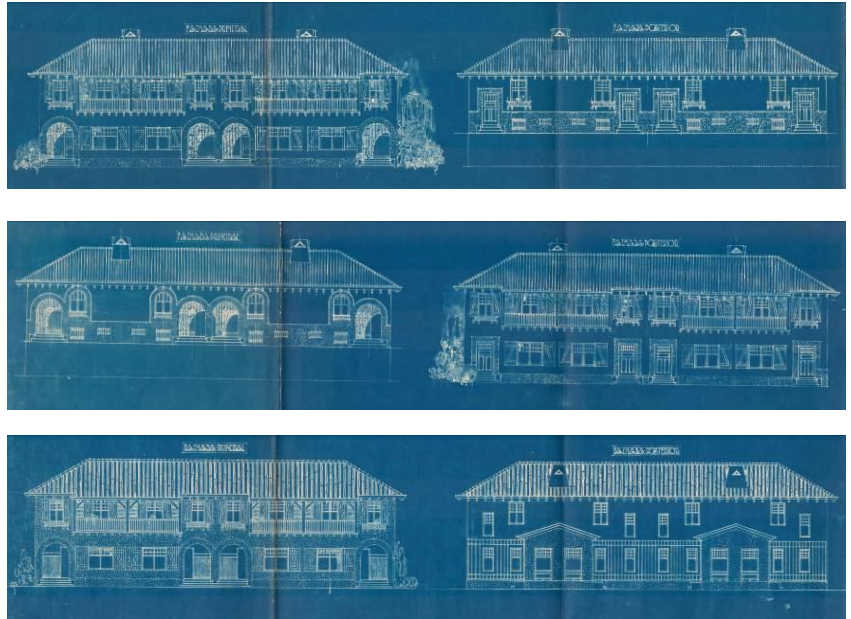
A, B eta C motako aurreko eta atzeko fatxadak hurrenez hurren
